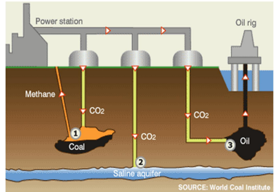
Hình: Mô hình công nghệ CCS, Photo © World Coal Institute
